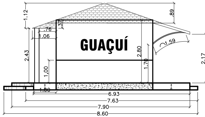
LATERAL NE ESCALA 1 / 100
