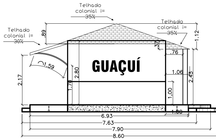
LATERAL NO ESCALA 1 / 100
