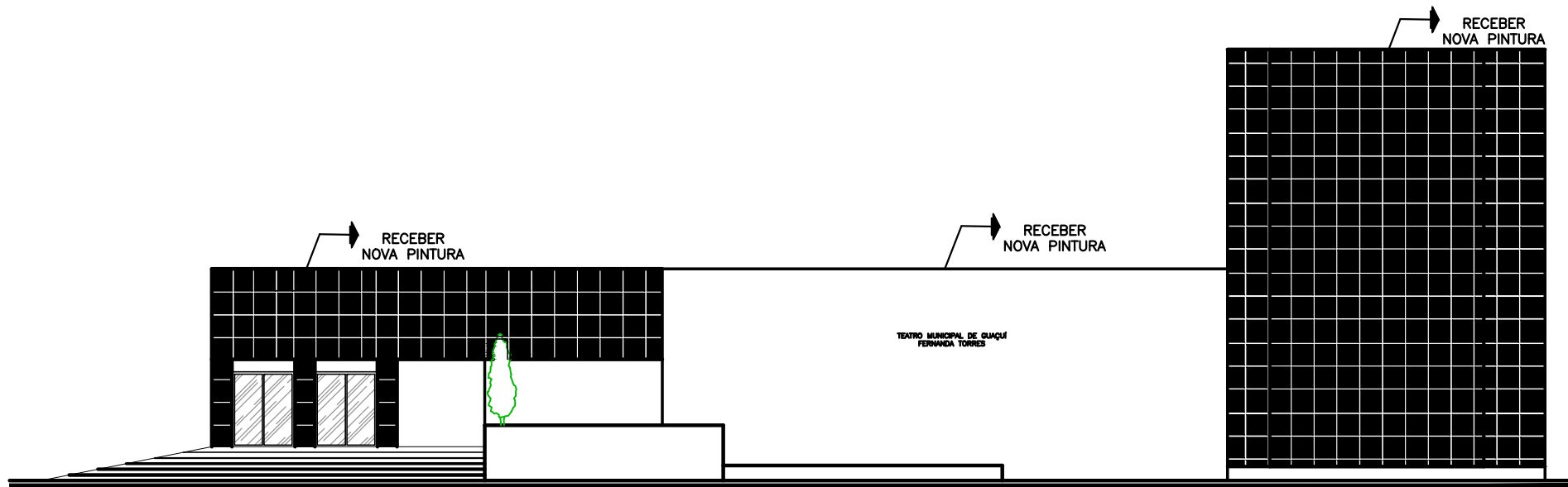
FACHADA FRONTAL esc 1:200
