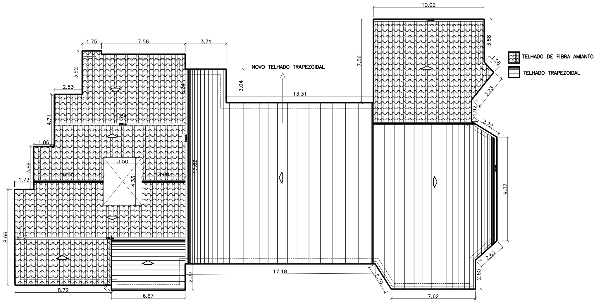
PLANTA DE COBERTURA esc 1:200
