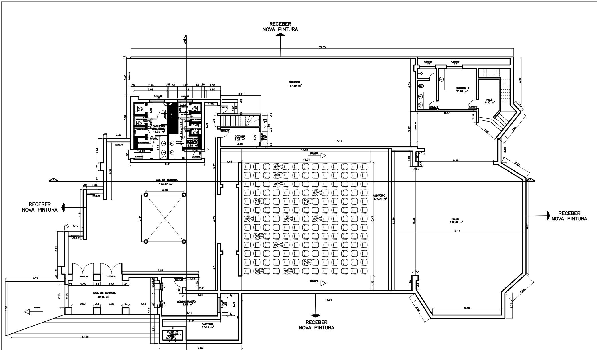
PLANTA BAIXA TÉRREO esc 1:200
